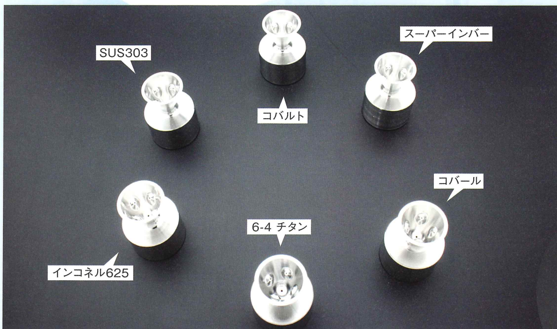
人工衛星燃料噴射ノズル 細穴Φ0.2mm×L2.0mm傾き45度
