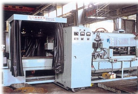
磁気探傷機
