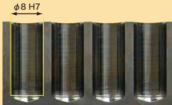
円筒度
