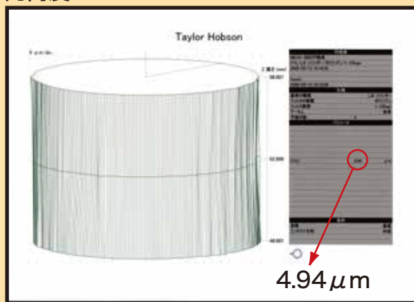
円筒度
