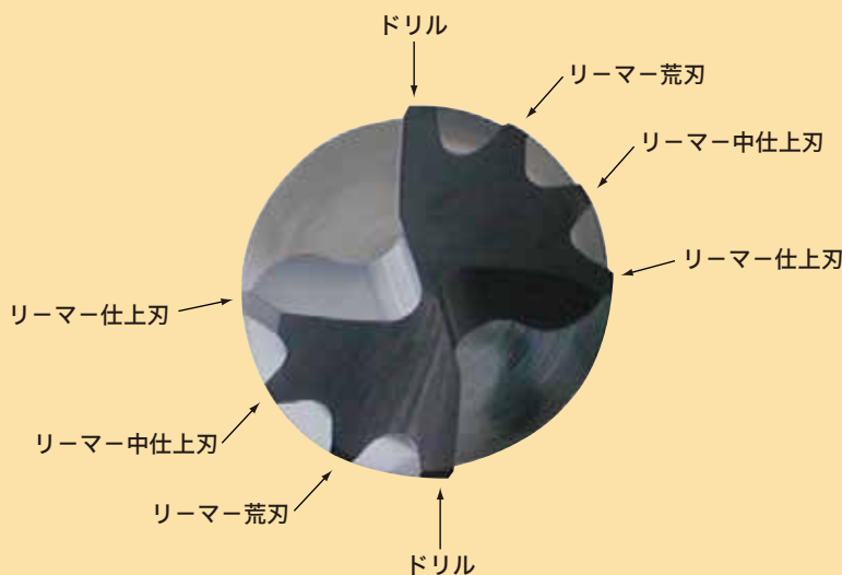
刃形状
