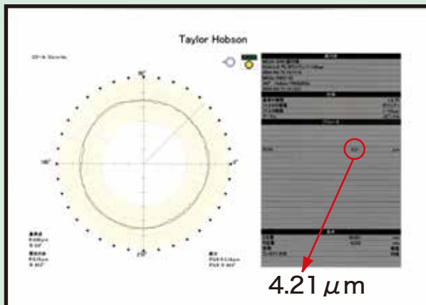
真円度
